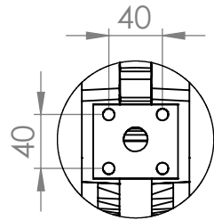
DETAIL A (LUMINAIRE INTERFACE)
