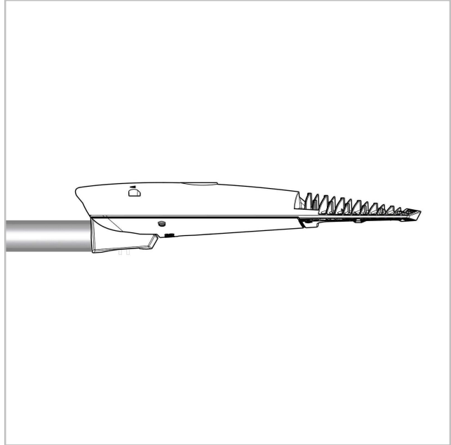
АКСІЯ 2 | Консольна насадка на Ø32 (через перехідник) або Ø42-60мм - кріплення 2xM10
